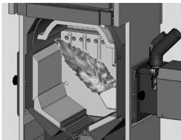
Brennerflamme, endend 1 - 3 cm vor der Gegenwand.
