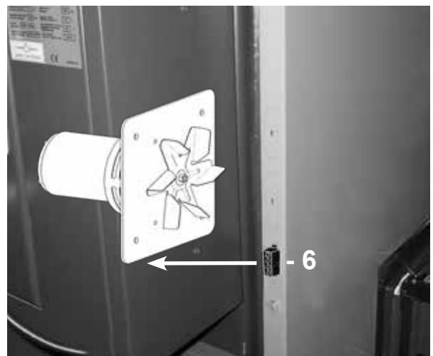
Steckverbindungen in der rechten Kesselabdeckung
