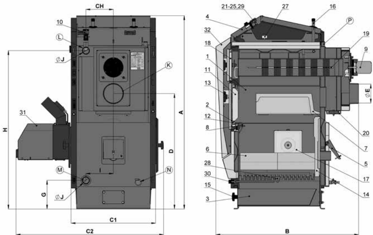
Querschnitt des Kessels P30, P40, P50
