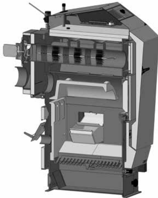
Kessel mit Saugzugventilator
