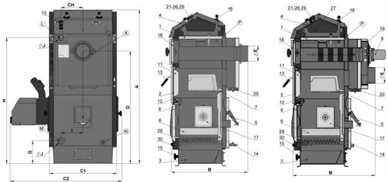
Querschnitt des Kessels P15, P20
